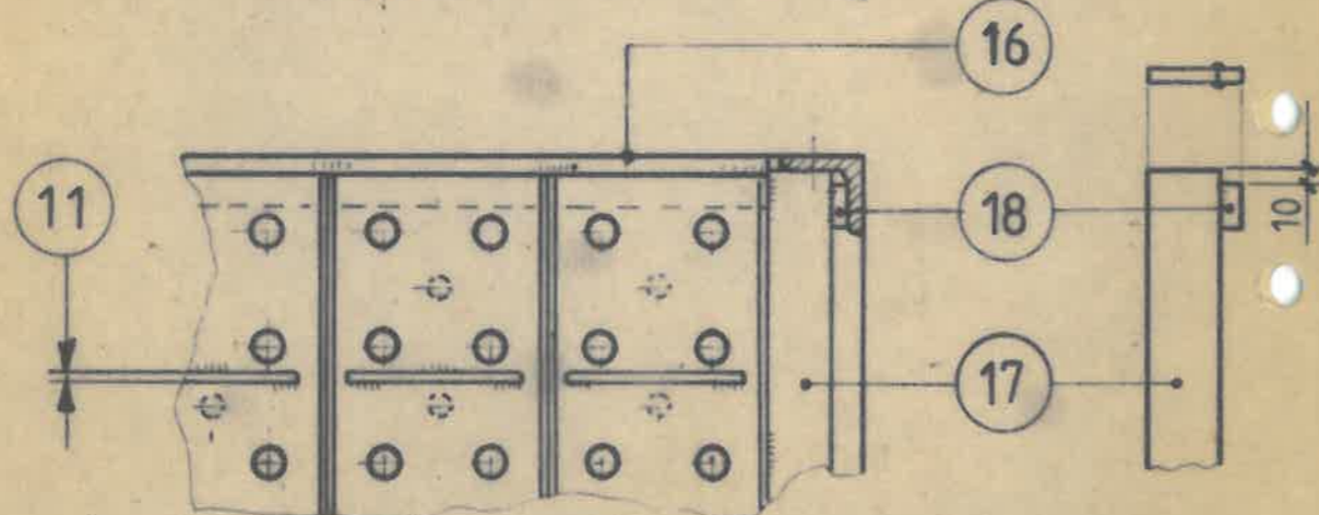
DOORSNEDE: A.A schaal 1:5
